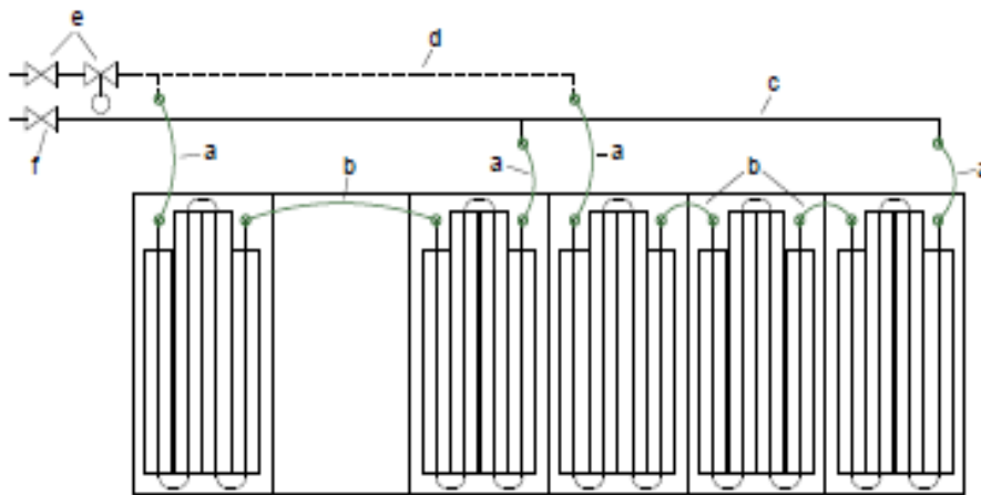
Bild 50 - Beispiel Anschluss aktiver Heiz- Kühldeckenplatten
