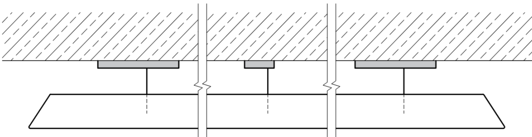
Bild 42 - Beispiel Thermoaktives Deckensegel (TABS)
