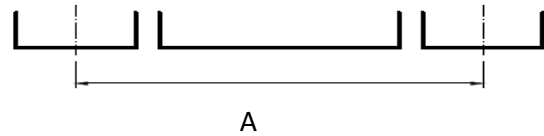
Bild 58 - Beispiel Achsmaß Bandrasterdecke
