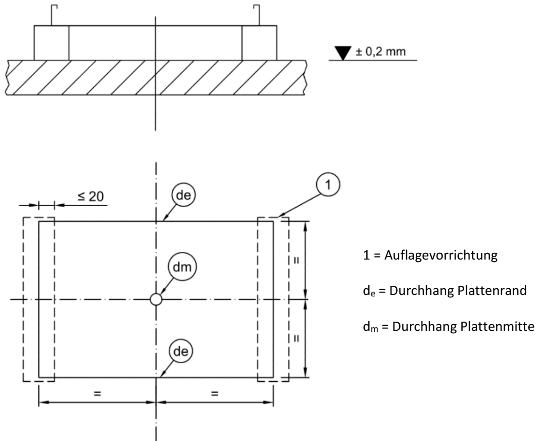
Bild 68 - Prüfung der Ebenheit von Metaldeckenplatten und Kassetten
