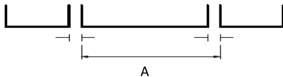
Bild 59 - Beispiel Modulmaß der Decklage
