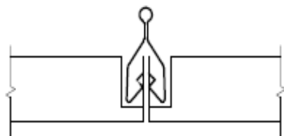
Bild 6 - Beispiel Klemmsystem mit verdecktem Klemmprofil
