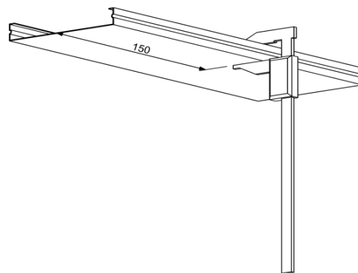
Bild 67 - Prüfung Kanthöhe Paneele Beispiel C-Kantung
