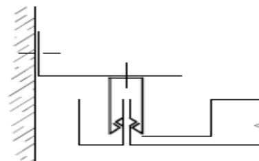
Bild 7 - Beispiel Klemmsystem mit Randwinkel
