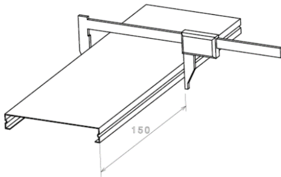
Bild 64 - Prüfung der Paneelbreite
