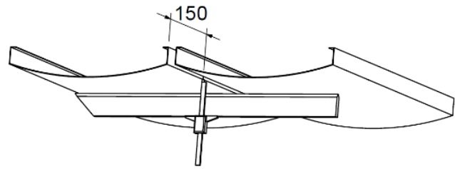
Bild 70 - Prüfung Ebenheit – Durchhang von Paneelen (konvex)
