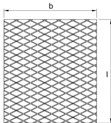
Bild 37 - Beispiel Streckgitterplatte Plattenlänge/ -breite
