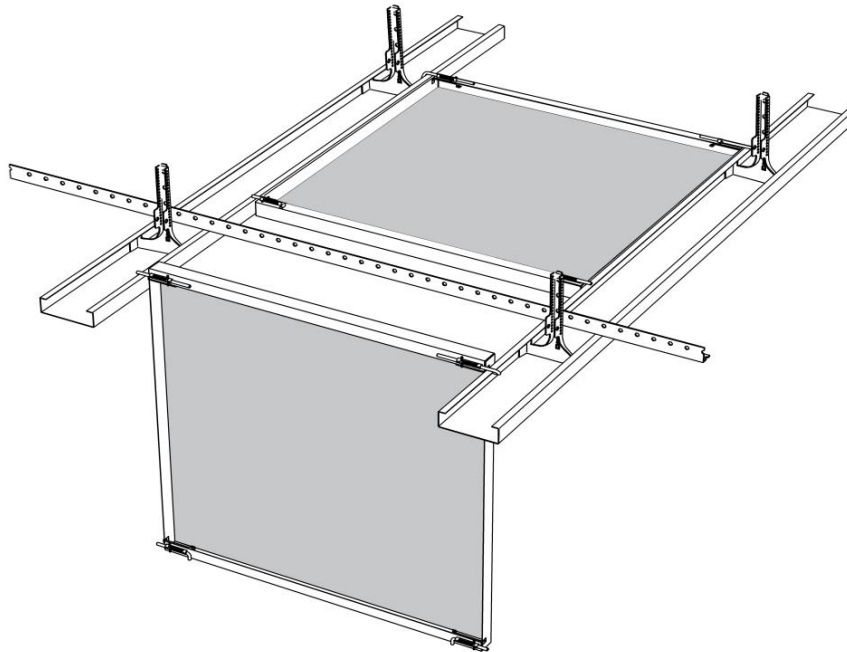
Bild 20 - Beispiel Bandasterdecke – Decklage abklappbar und verschiebbar
