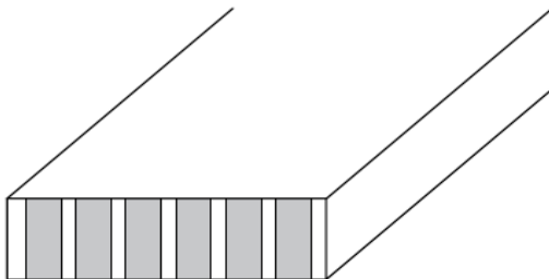
Bild 40 - Beispiel Verbundelement bestehend aus Aluminiumwabenkern mit beidseitig verklebten Metallblech
