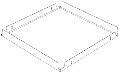
Bild 16 - Beispiel Klemmkassette 4-seitig mit L-Kante
