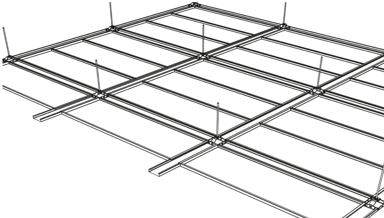
Bild 13 - Beispiel Kreuzbandrasterdecke mit Knotenpunkt
