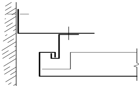
Bild 4 - Beispiel Einhängesystem mit Einhängeprofil und Randprofil
