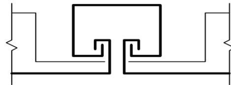
Bild 3 - Beispiel Einhängesystem mit Doppelseinhängeprofil
