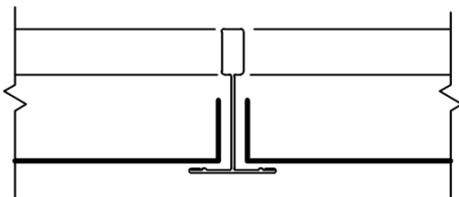
Bild 18 – Beispiel Aufgelegtes System T-Profilkonstruktion mit aufgelegter Platte
