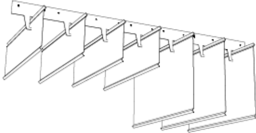
Bild 28 - Beispiel Vertikallamellendecke mit Tragschiene und einwandigen Lamellen
