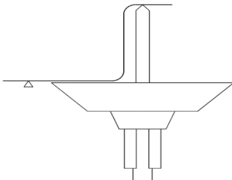
Bild 66 - Prüfung Kanthöhe Beispiel Z-Kantung nach aussen
