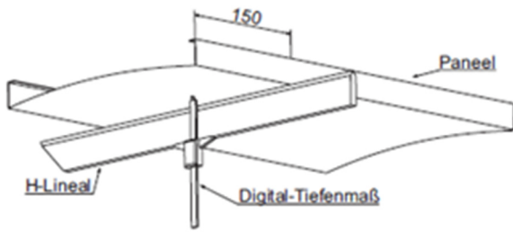
Bild 69 - Prüfung der Ebenheit – Wölbung von Paneelen
