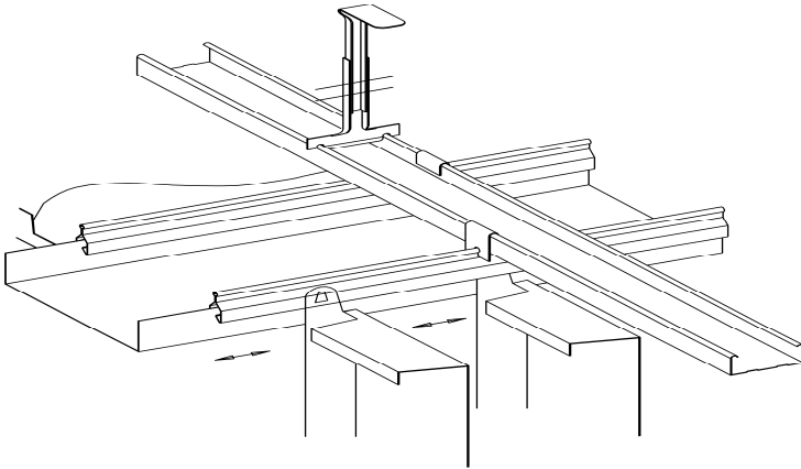
Bild 8 - Beispiel Klemm – Klappsystem Klemmkassette mit Haltetasche
