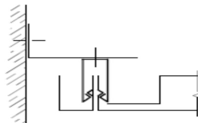
Bild 7 - Beispiel Decklage im Klemmsystem mit Randwinkel
