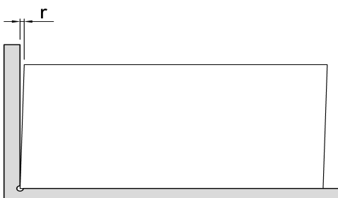
Bild 72 - Prüfung der Rechtwinkligkeit
