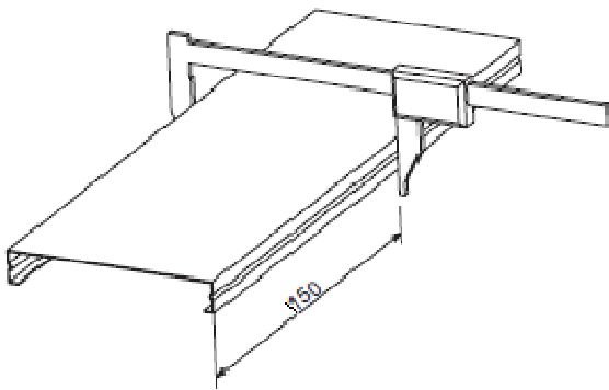
Bild 64 - Prüfung der Breite bei Paneelen
