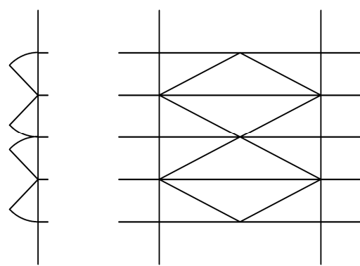
Bild 22 - Beispiel Klapprichtungen über die Längsachse der Decklage - Richtung zueinander
