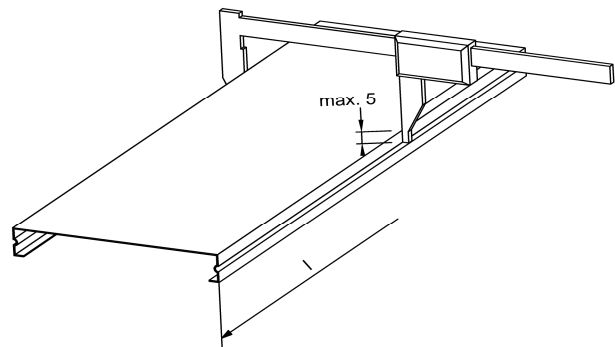
Bild 65 - Prüfung der Breite/Länge bei einer Metaldeckenplatte und -kassette
