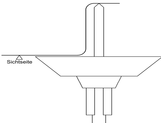
Bild 66 - Prüfung der Kanthöhe Beispiel Z-Kantung nach aussen
