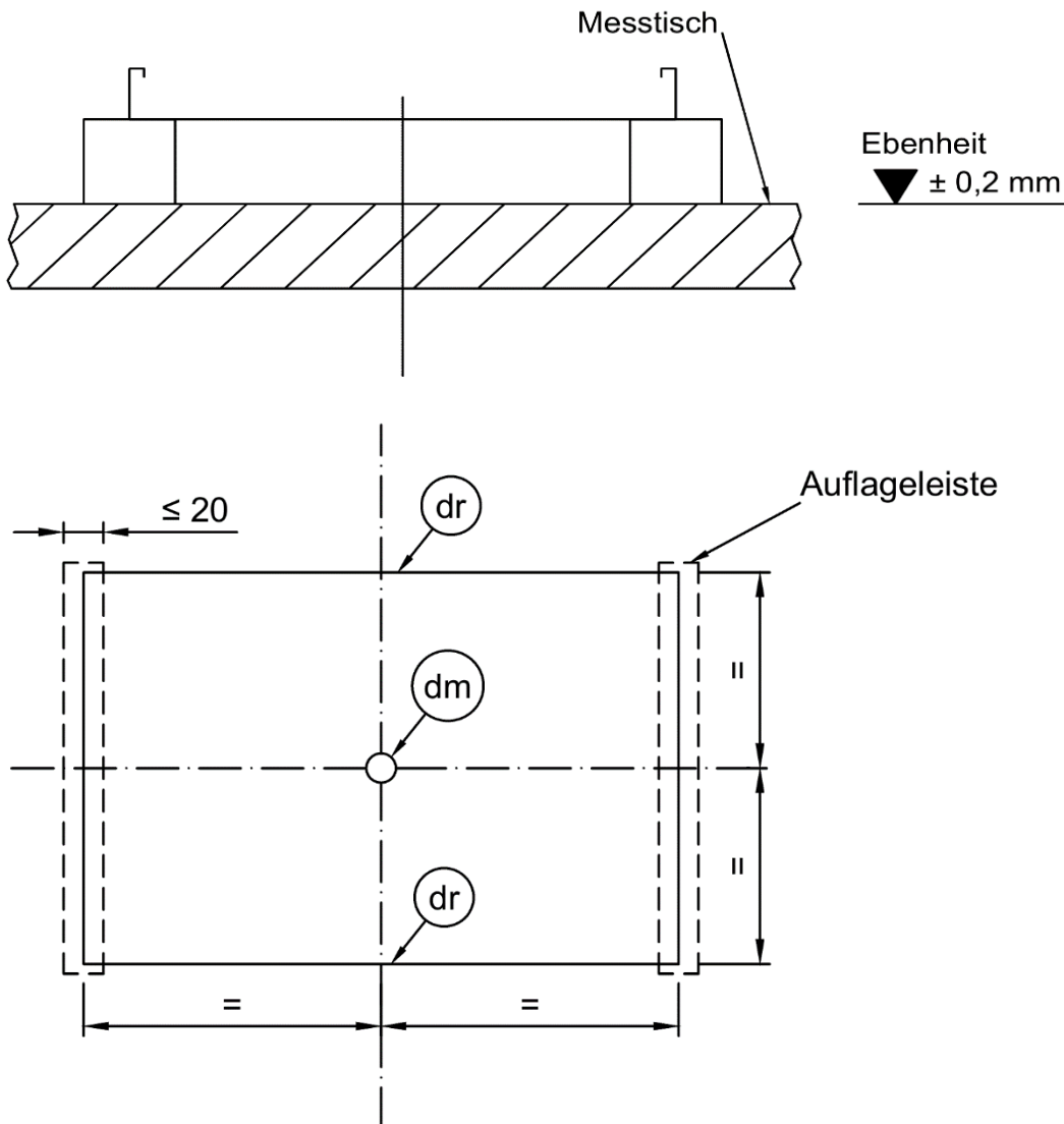
Bild 68 - Prüfung der Ebenheit bei Metalldeckenplatten und Kassetten
