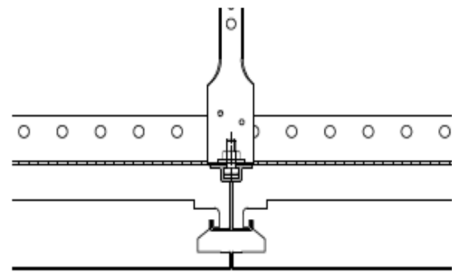
Bild 5 - Beispiel Decklage im Einhängesystem mit T-Ein角度
