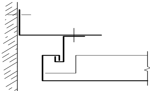
Bild 4 - Beispiel Decklage im Einhängesystem mit Einhängeprofil und Randprofil
