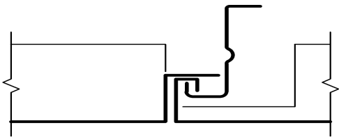
Bild 2 - Beispiel Decklage im Einhängesystem mit Einhängeprofil
