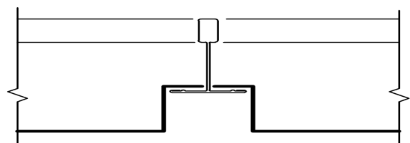
Bild 19 - Beispiel Aufgelegtes System T-Profilkonstruktion mit eingeleger Platte
