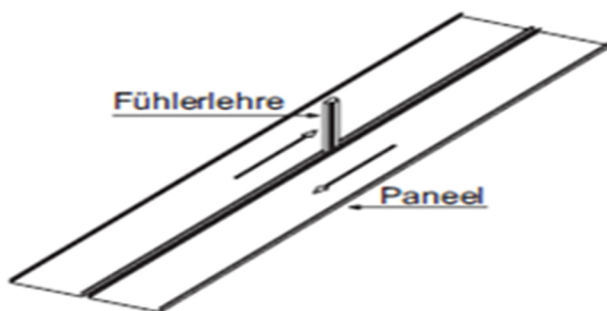
Bild 71 - Prüfung der Säbeligkeit von Paneelen
