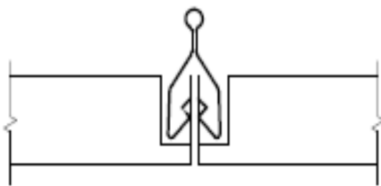
Bild 6 - Beispiel Decklage im Klemmsystem mit verdecktem Klemmprofil
