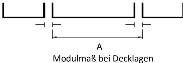
Bild 59 - Beispiel Modulmaß der Decklage
