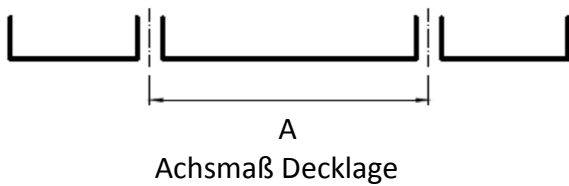
Bild 57 - Beispiel Achsmaß der Decklagen
