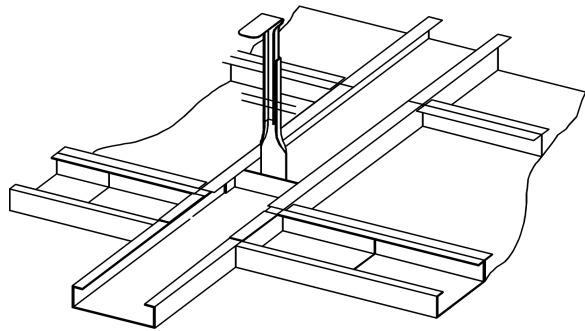
Bild 12 - Beispiel Kreuzbandrasterdecke Abhängung
