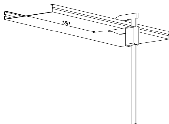
Bild 67 - Prüfung der Kanthöhe einer Paneele Beispiel C-Kantung nach innen
