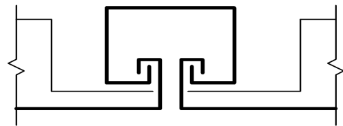
Bild 3 - Beispiel Decklage im Einhängesystem mit Doppelsein角度
