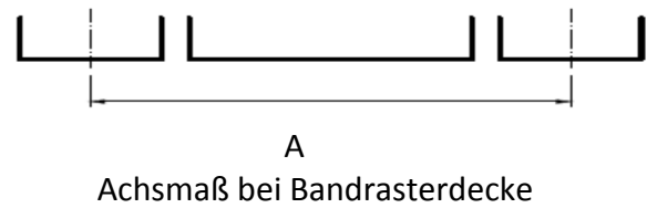
Bild 58 - Beispiel Achsmaß Bandrasterdecke
