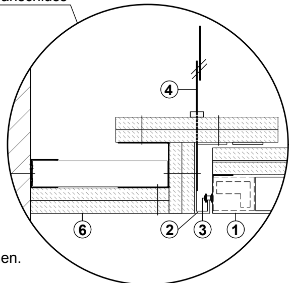
Schnitt Wandanschluss
